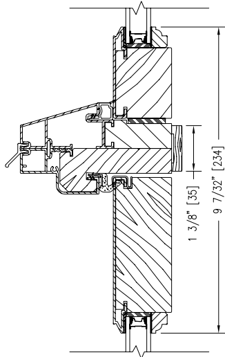
INSWING TRANSOM OVER INSWING DOOR
